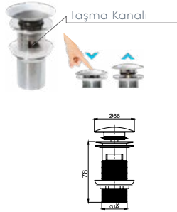
Yuvarlak Lavabo Süzgeci Aç/Kapa
